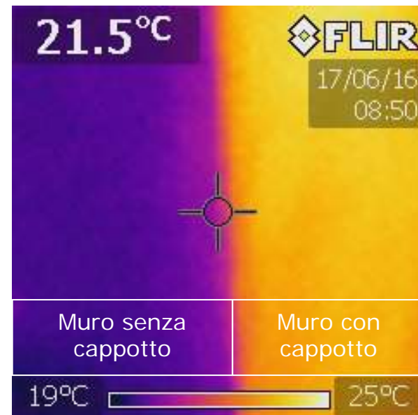
Termografia
