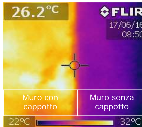
Termografia
