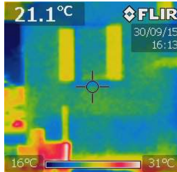
Termografia prima dell'applicazione
